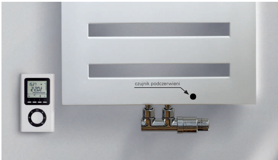
Grzejniki łazienkowe Premium MIX zasilany wodno-elektrycznie z elektronicznym regulatorem oraz czujnikiem podczerwieni zintegrowanym w korpus grzejnika
